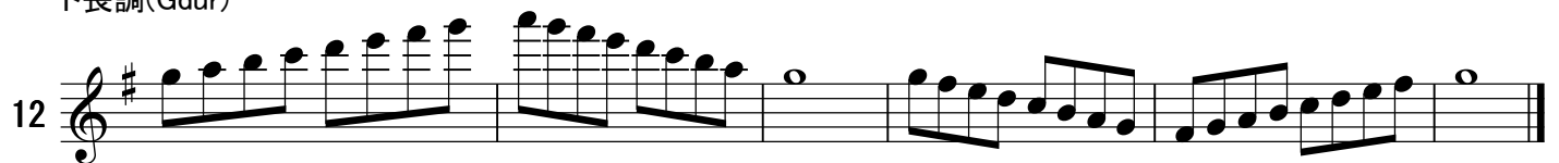
ト長調(Gdur)
